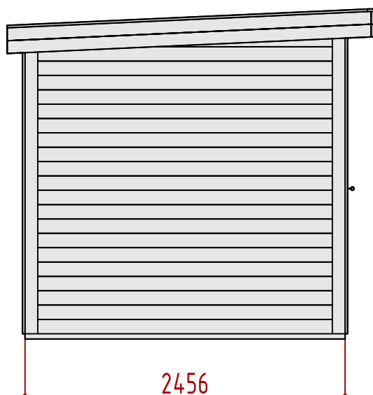
SIDE FASADE
